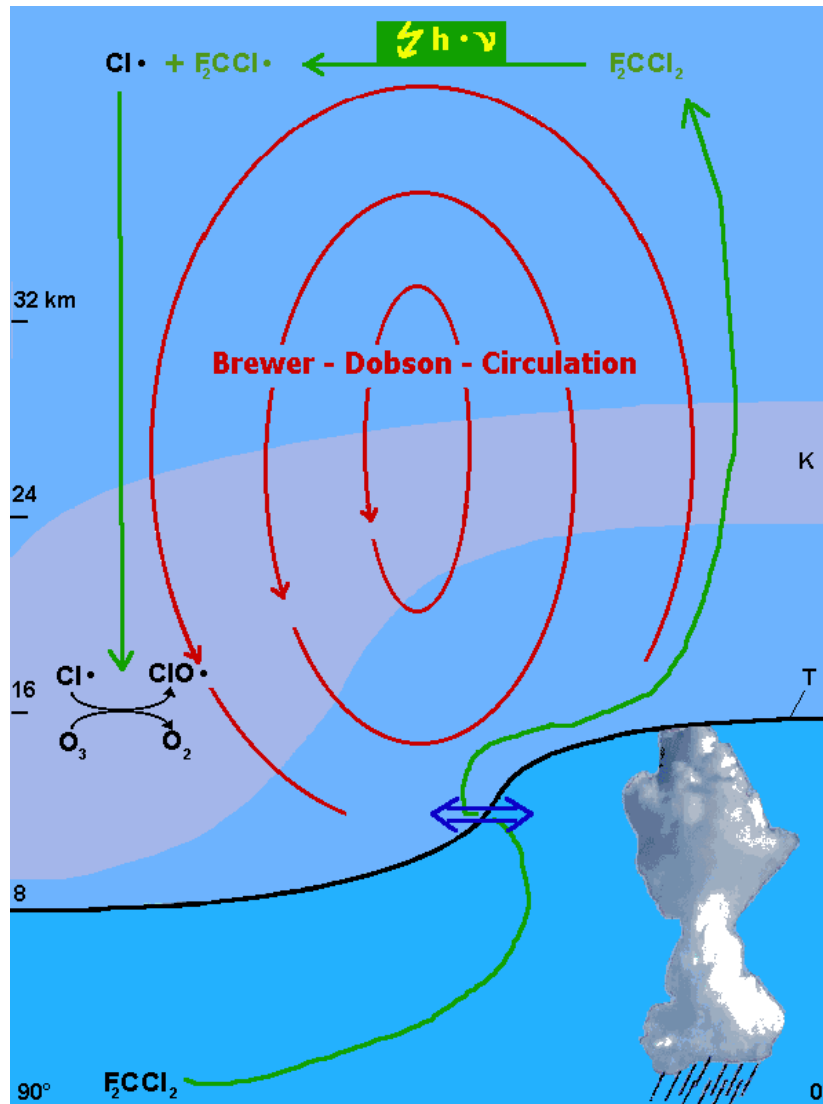
Figure 2: Strati dell'atmosfera dall'equatore al polo nord (T: tropopausa; K: area della stratosfera con alte concentrazioni di ozono (>16 DU / km))
