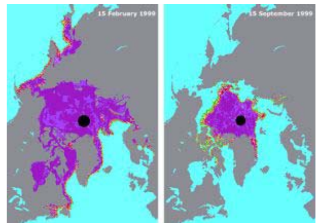
Seeeis um den Nordpol (in violett) im Februar (links) und im September 1999 (rechts)
